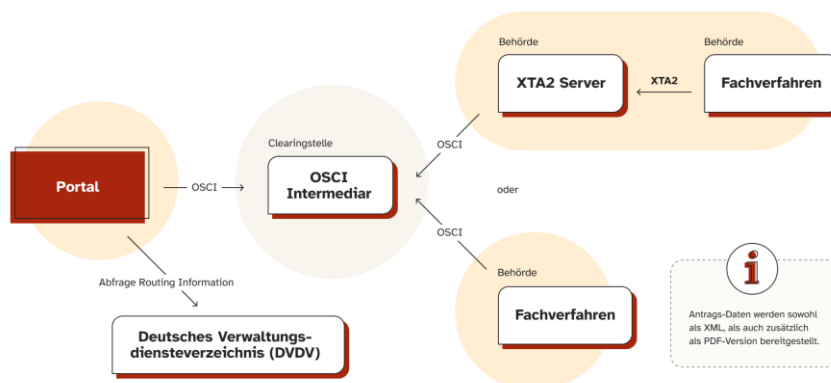
Abbildung 5: Anbindungsvariante 1: Direkte Fachverfahrensanbindung
